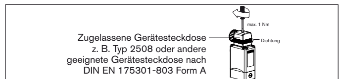
Bild 3: Elektrischer Anschluss der Gerätesteckdose
