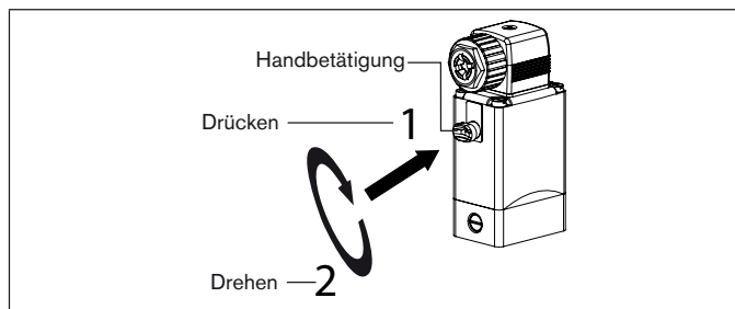
Bild 2: Handbetätigung
