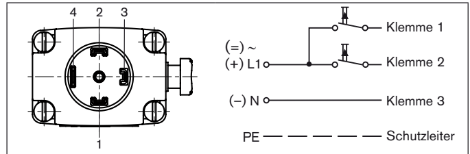
Bild 4: Elektrischer Anschluss - Impulsausführung (CF 02)
