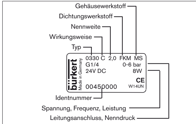
Bild 1: Beschreibung des Typschilds (Beispiel)
