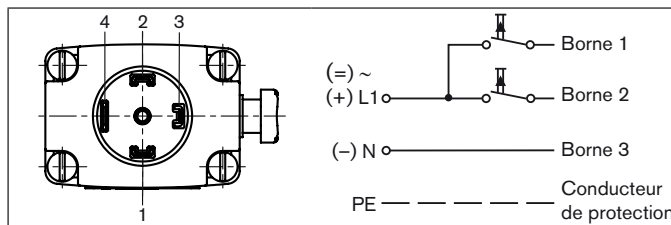
Fig. 4 : Raccordement électrique - Version à impulsion (CF 02)
