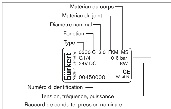
Fig. 1 : Description de la plaque signalétique (exemple)
